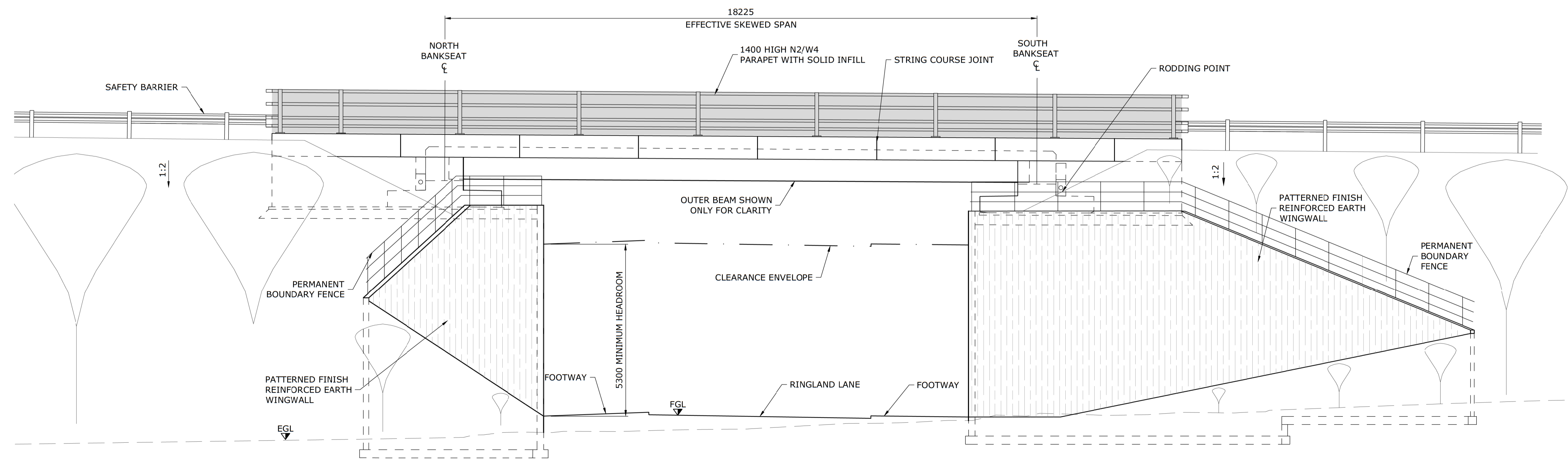
ELEVATION A-A 1:75
